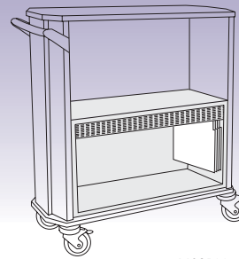
64021** Wide, 1 Quando A4/folio suspension files
